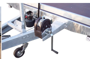
Torreta con cabrestante 1600kg. Plataformas TOPLINE 620/622/630/632
